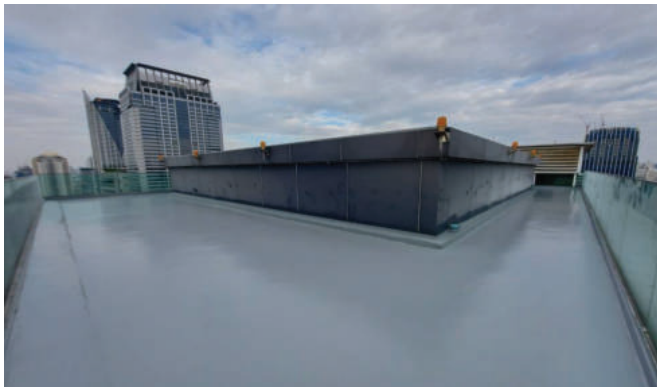
งานกันซึมดาดฟ้าระบบโพรียูรีเทน 3 mm. 1,300 ตรม. สำนักงานตำรวจแห่งชาติ
